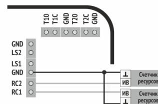
Схема подключения счетчиков воды:
